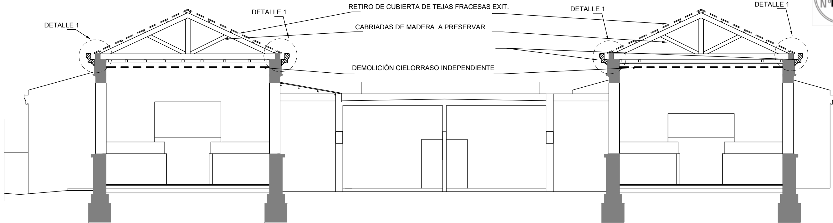
CORTE A-A
