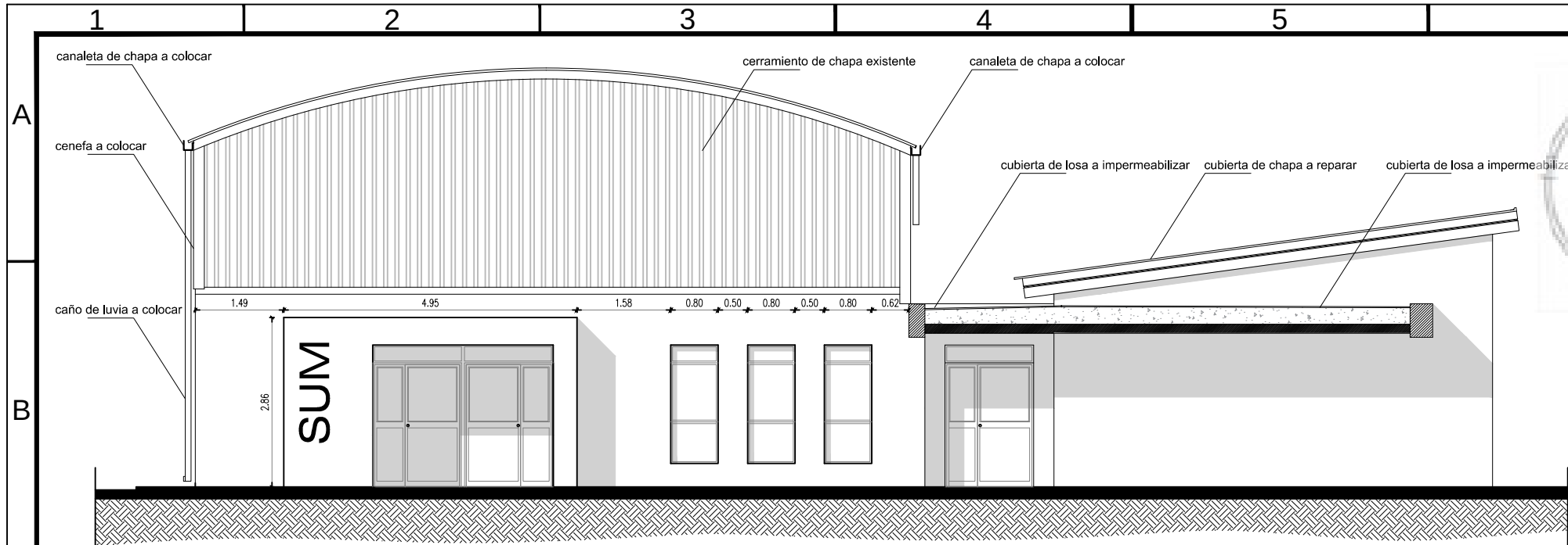
VISTA OESTE
