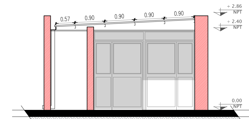
CORTE C-C
