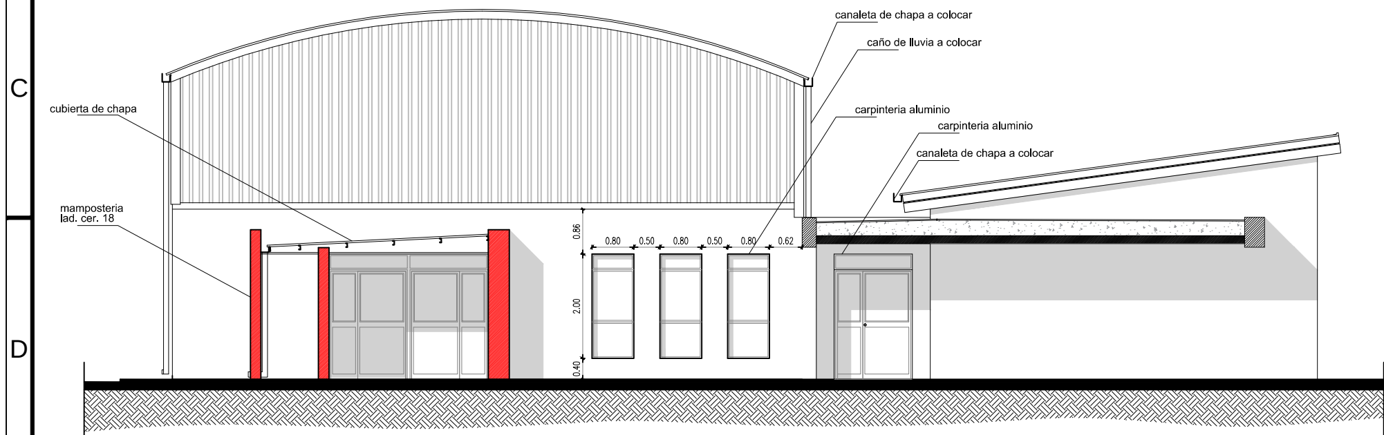
CORTE A-A
