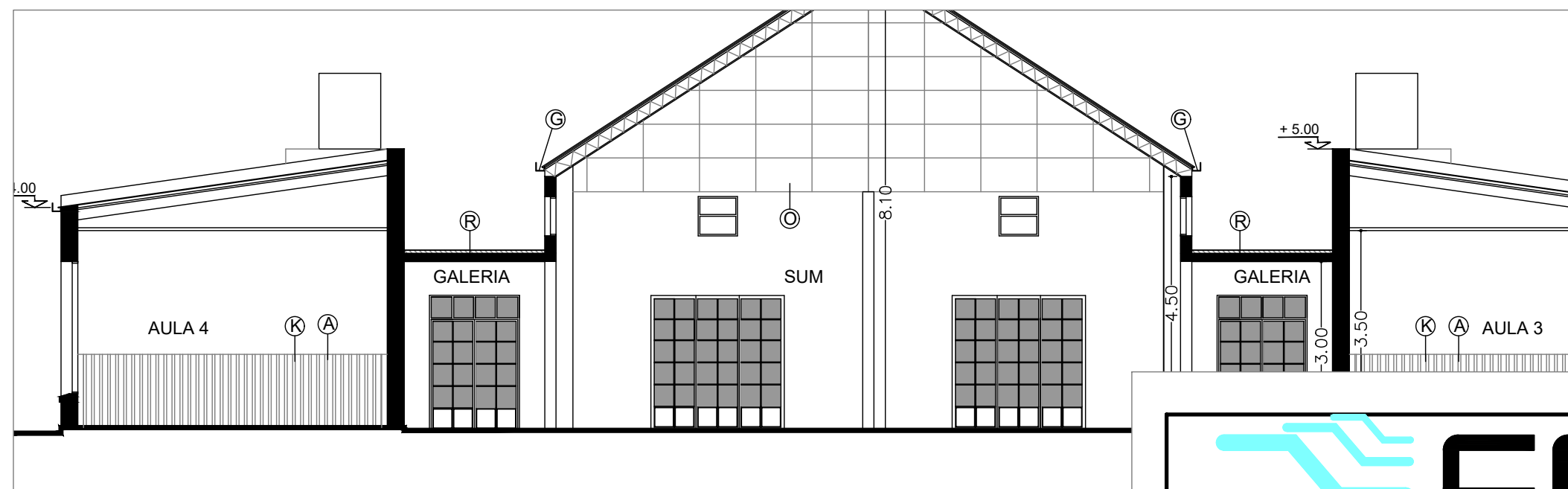
CORTE A-A (EXISTENTE) - ESC. 1:100
