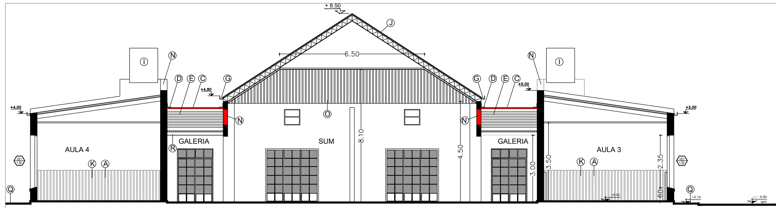
CORTE A-A (CON INTERVENCIÓN) - ESC. 1:100
