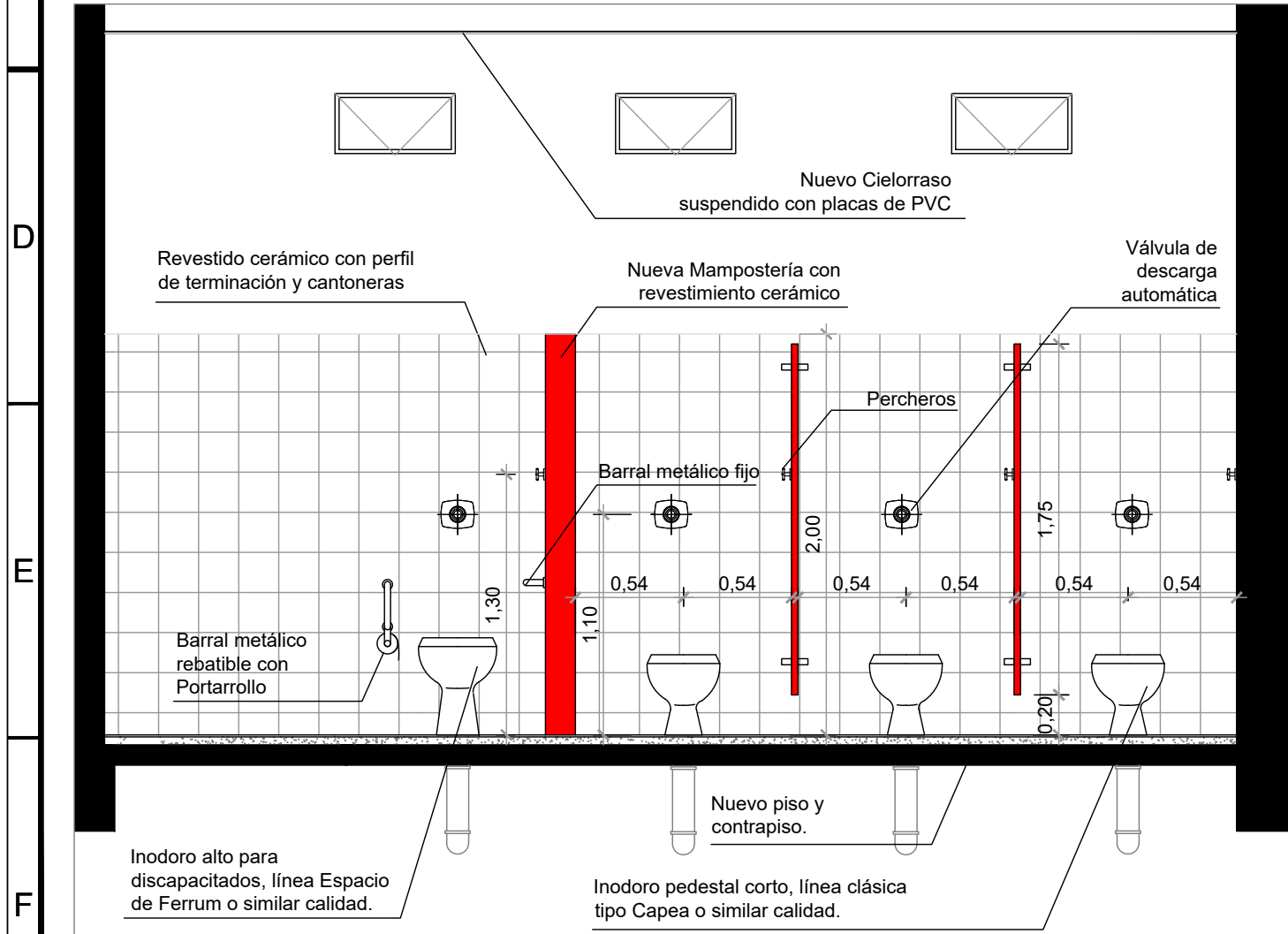
CORTE BOX SANITARIOS
