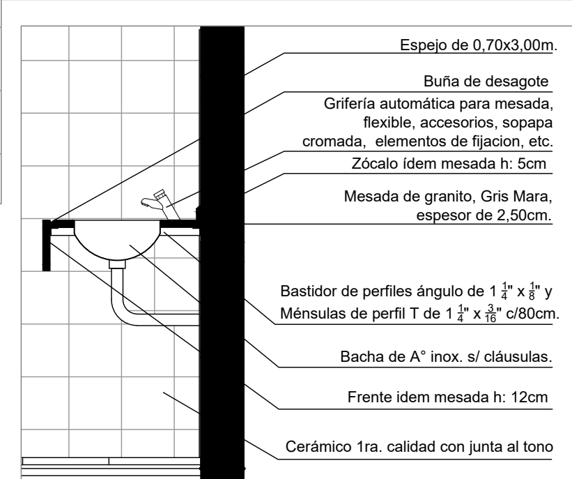
CORTE MESADA SANITARIOS
