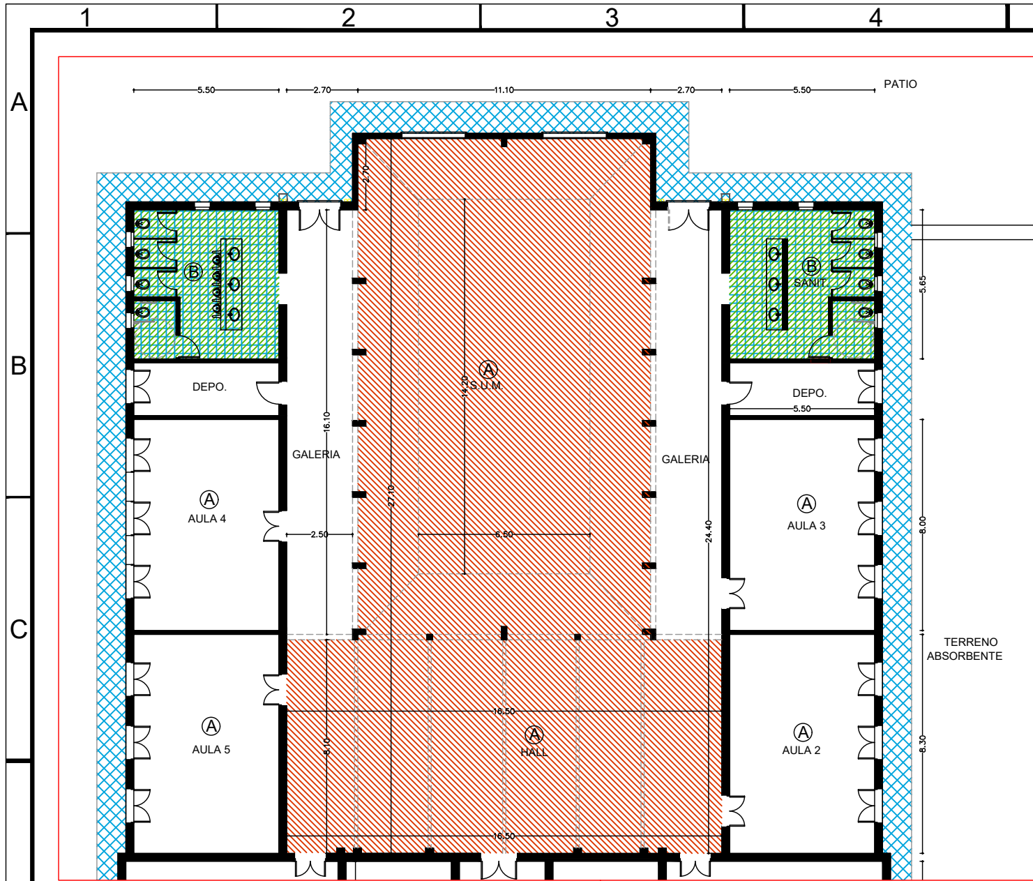
PLANTA SECTOR ESTE - ESC. 1:200
