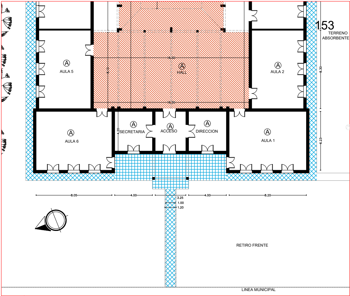
PLANTA SECTOR OESTE ESC. 1:200
