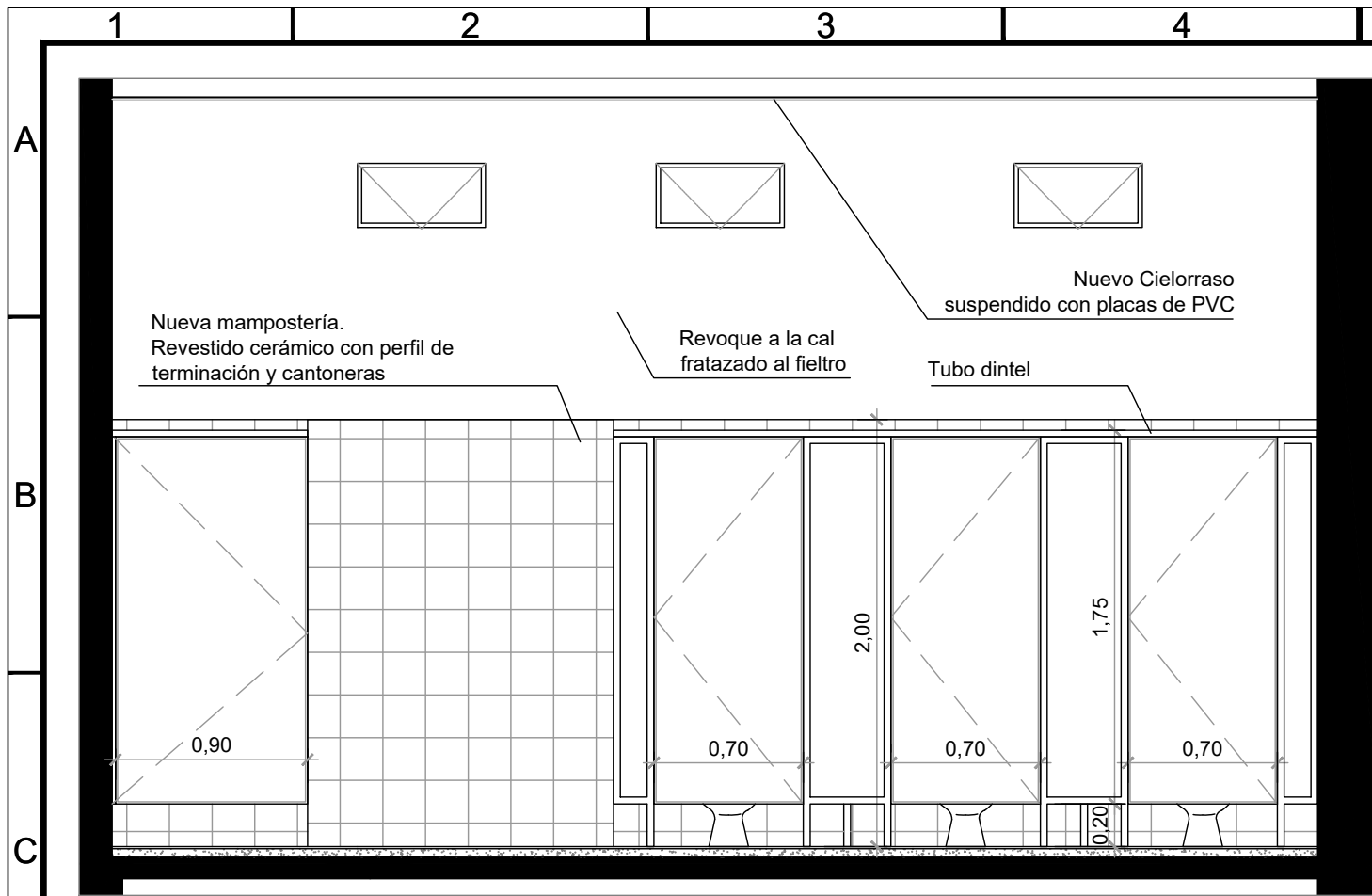
VISTA FRETE BOX SANITARIOS
