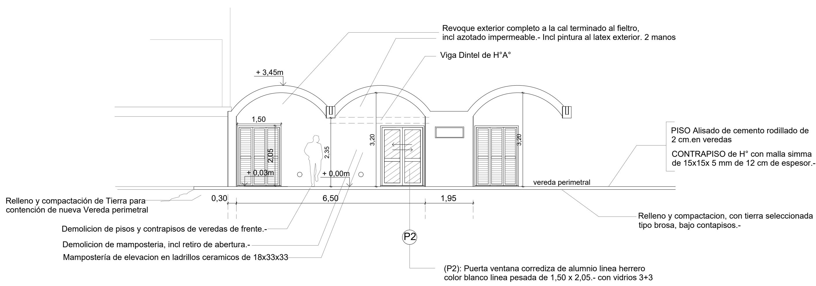
VISTA FRONTAL 5-5 esc 1:75
