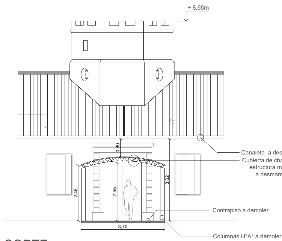
CORTE GALERÍA DE INGRESO
