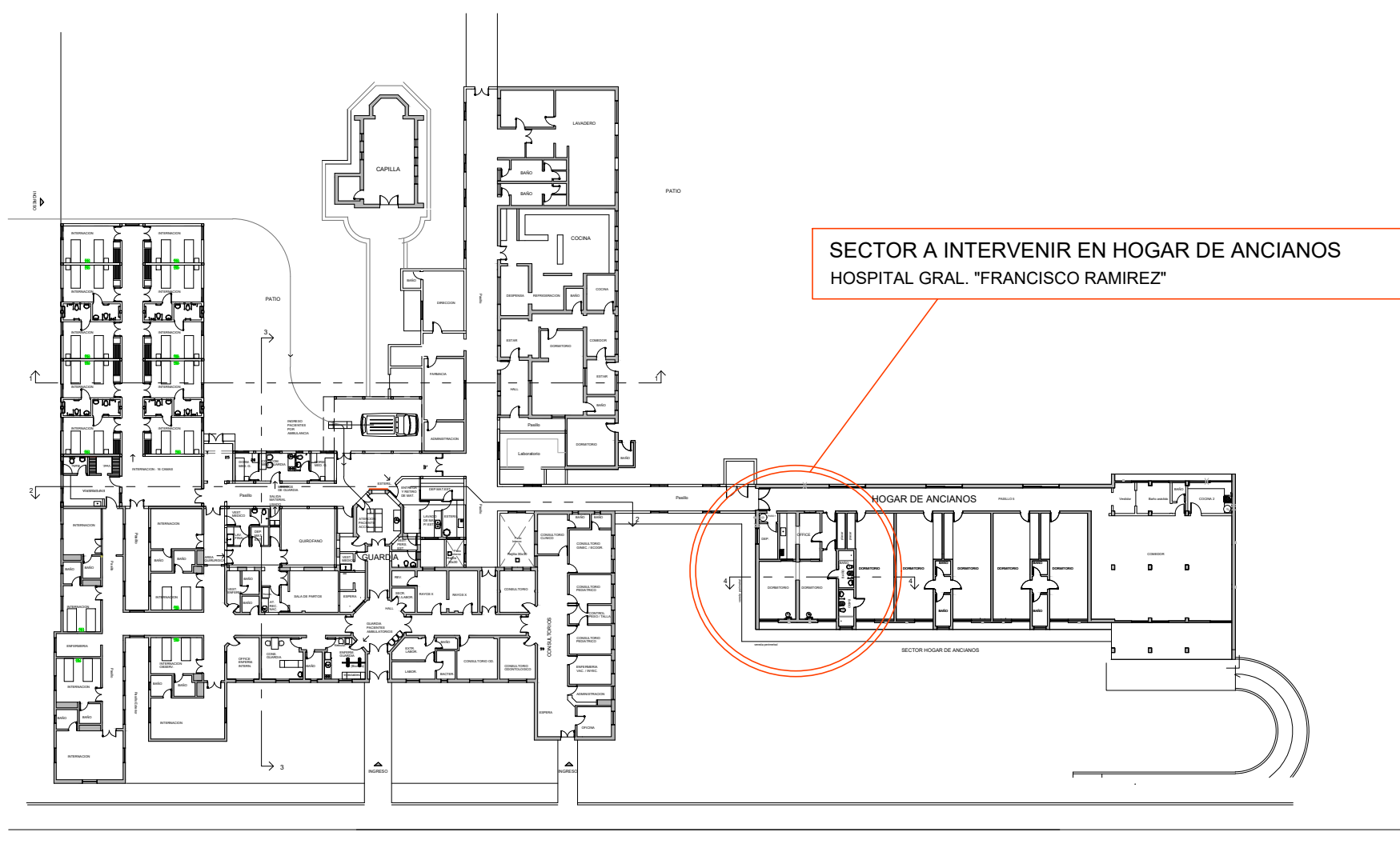
PLANTA (RELEVAMIENTO FOTOGRÁFICO) SECTOR HOGAR DE ANCIANOS
