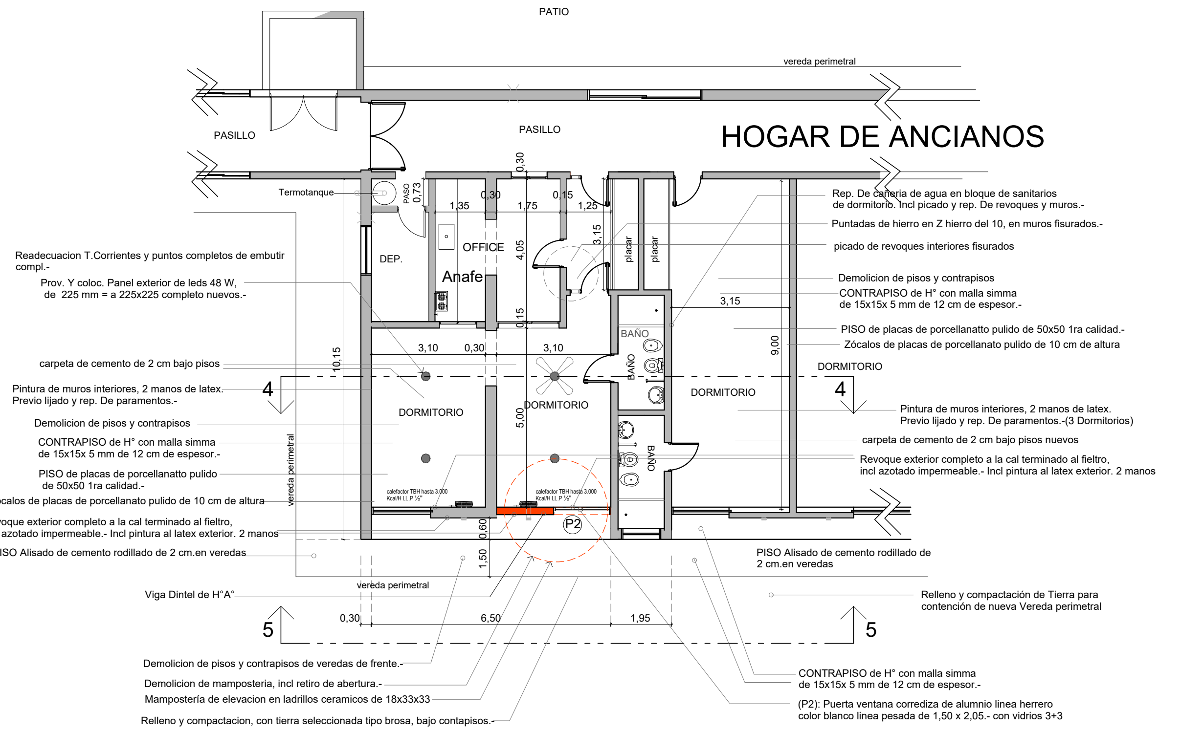
PLANTA SECTOR A INTERVENIR esc 1:100
