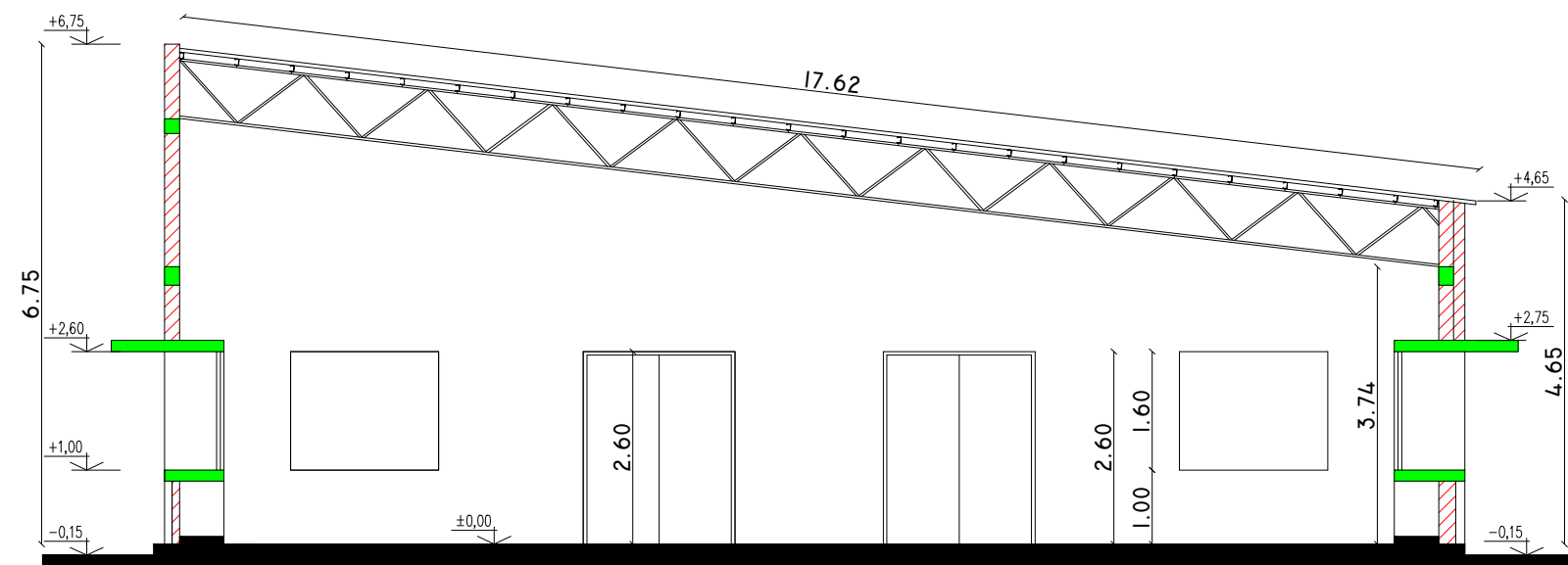
CORTE A-A
