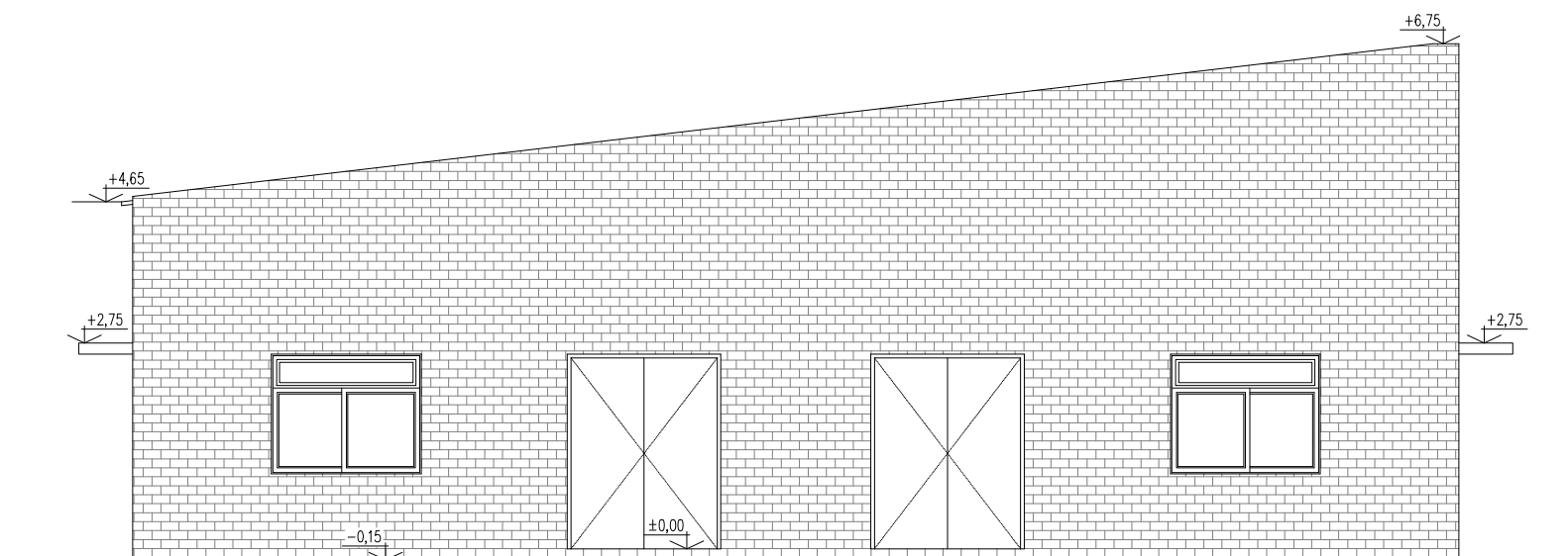
FACHADA NORTE
