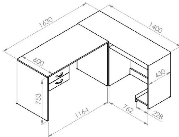
Esquema de medidas
