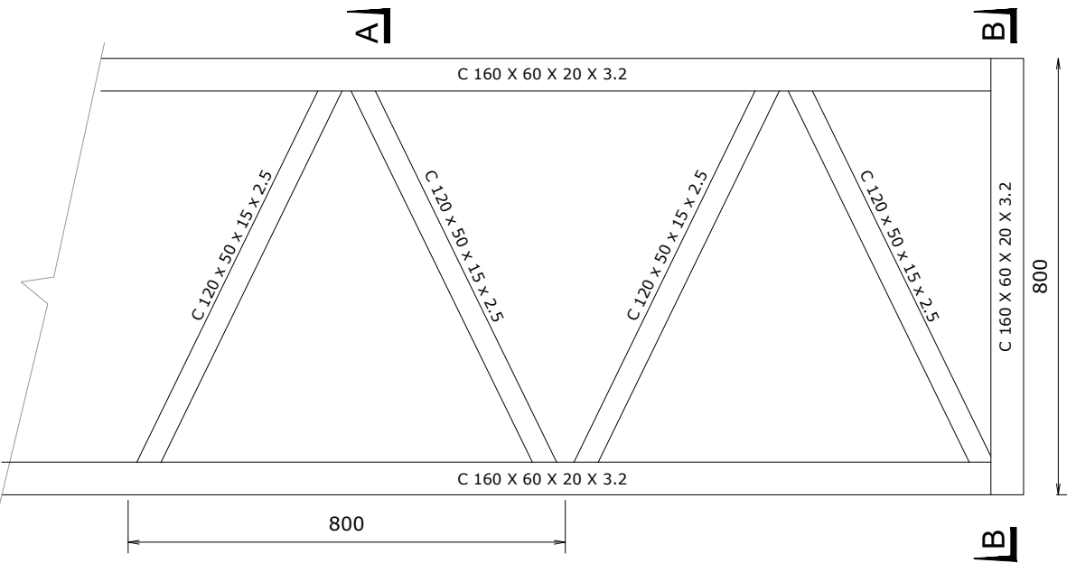
Celosías laterales de VR1
