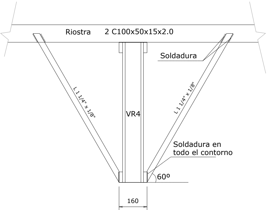
Detalle Tornapunta
