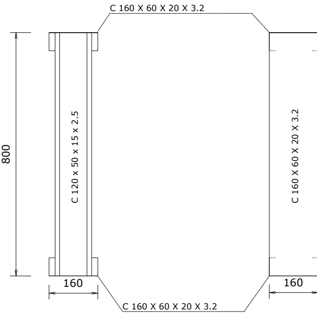
SECCIÓN A-A
